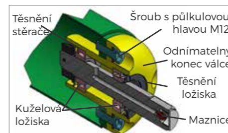
Vnitřní ložiska válce (na všech strojích Major Swift a Synergy)
